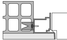
INSTALLAZIONE PER PARETE IN MURATURA
