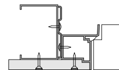
INSTALLAZIONE PER PARETE IN CARTONGESSO
