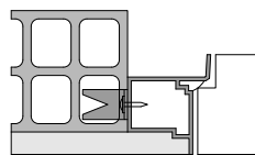
INSTALLAZIONE PER PARETE IN MURATURA
