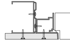
INSTALLAZIONE PER PARETE IN CARTONGESSO
